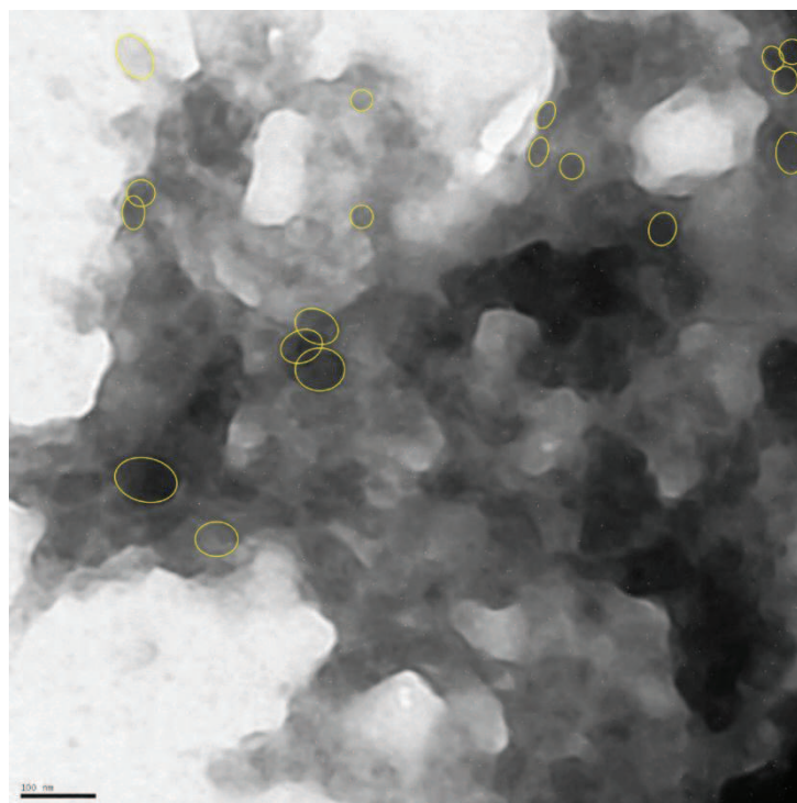
Figura 10: Micrografia da microscopia eletrônica de transmissão, escala de 100 nm.
