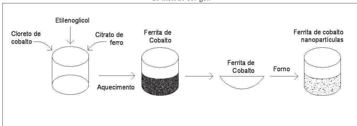
Figura 6: Demonstração esquemática dos compostos e procedimento utilizados para síntese de NPFC's através do método sol-gel.
