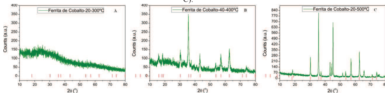
Figura 7: Difratograma de raios X nas diferentes temperaturas de síntese de NPFC's (A-300°, B-400° e C-500° C).
